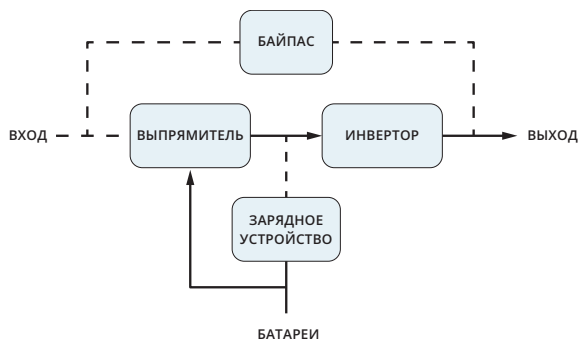
Рисунок 2.6. Режим работы от АКБ
